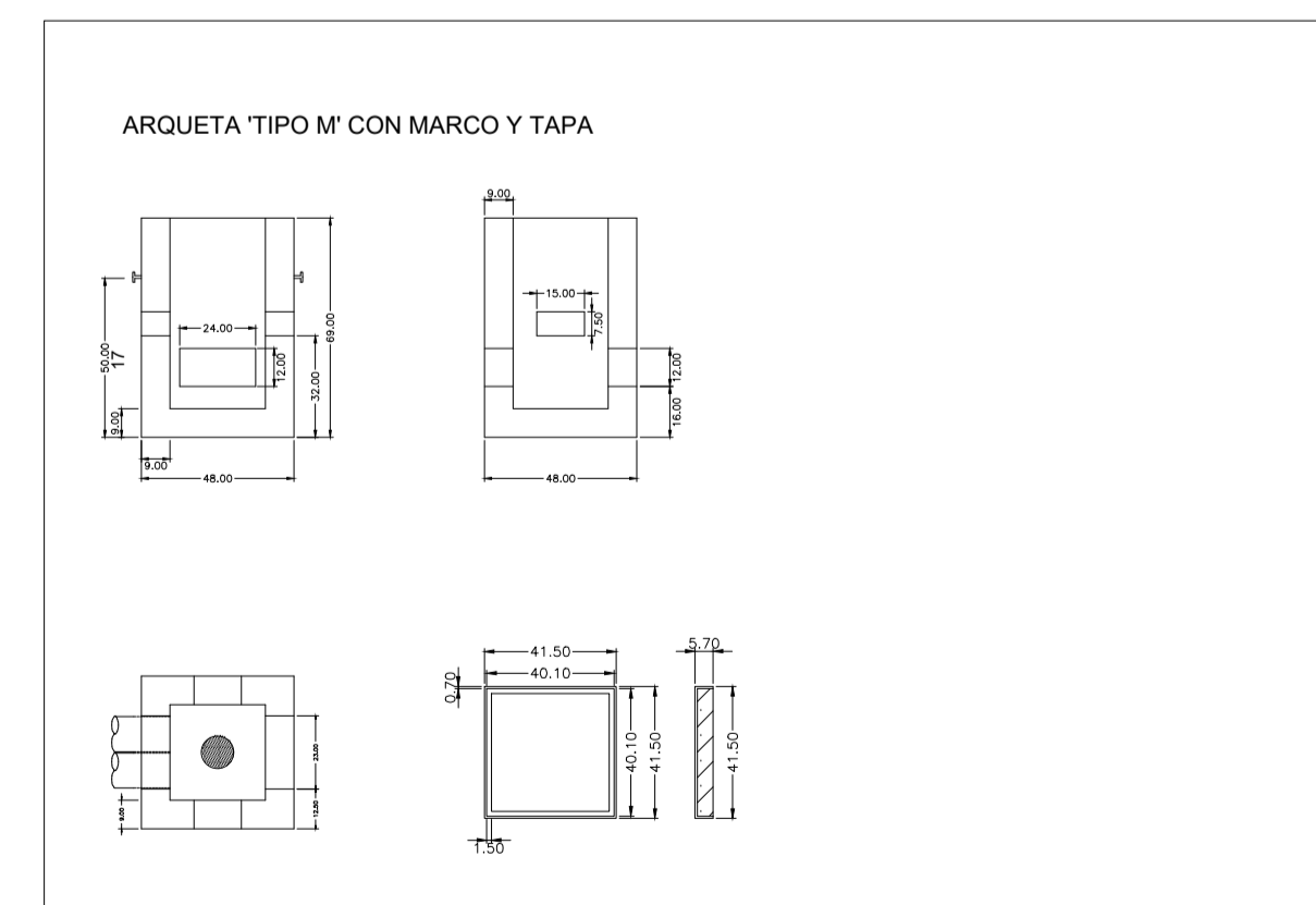
DETALLES TELECOMUNICACIONES
